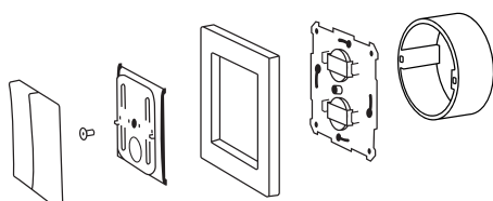
Montage an der Außenseite einer Gerätedose mit Schrauben
