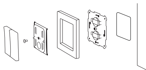
Montage mit beiliegendem Klebeband an einer Wand
